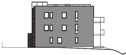
FASADE MOT NORD-VEST
