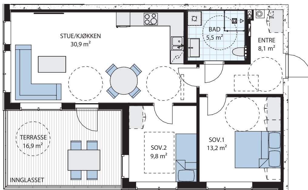
Målestokk 1:100
